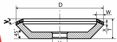
12V5-45° D*T*W*X*V*H
