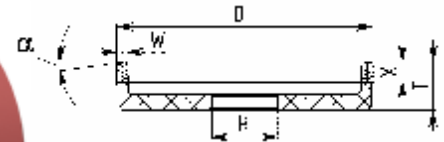
6A2 D*W*X*T*H*α°
