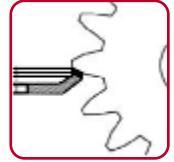
Заточка долбляка
